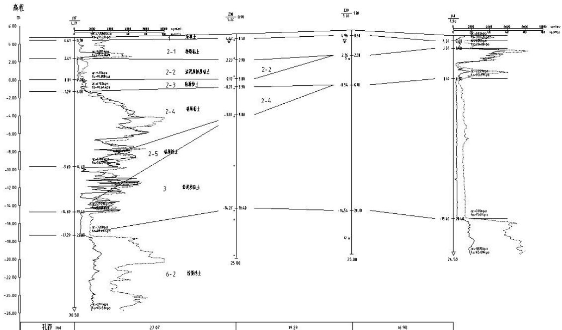
图3.1-1 区域典型地质剖面图
